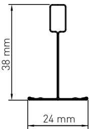
Hoofdprofiel
