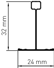
Tussenprofiel
