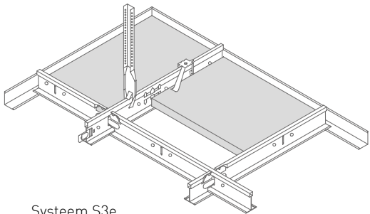
Systeem S3e
