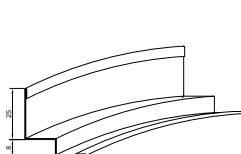
Nr. 50/15 G Contura wandprofiel
