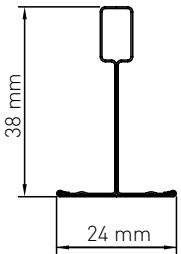
Tussenprofiel
