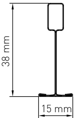
Hoofdprofiel
