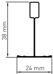
Hoofdprofiel
