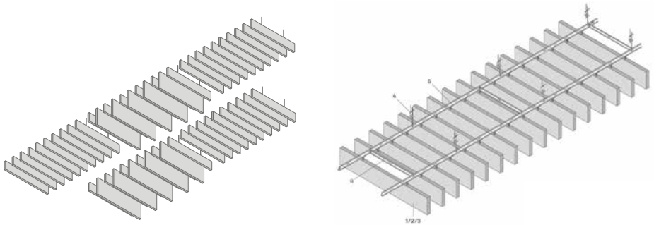
PER BAFFLE MET STOKSCHROEF MET S3 SYSTEEM
