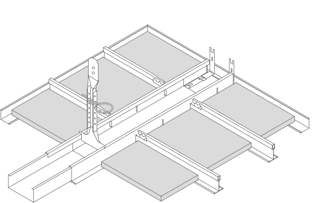
Systeem S18 S18d bandraster plafond met lange inleg panelen
