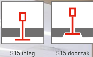
S15 inleg S15 doorzak
