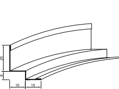
Nr. 50/15 G Contura wandprofiel
