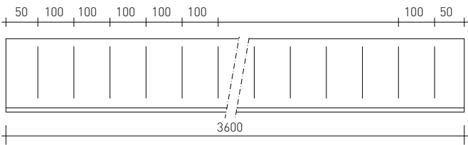
Bandraster ongesleufd BR100
