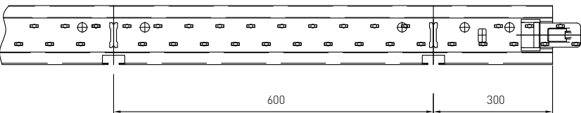
OWAline T 1200 en 600
