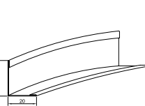
Nr. 50 G Wandprofiel
