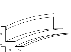
Nr. 50/15 G Contura wandprofiel
