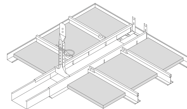
Systeem S18 S18d bandraster plafond met lange inleg panelen
