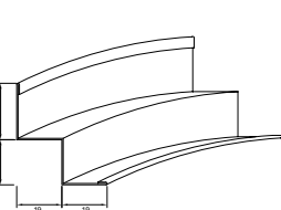
Nr. 56/20 Niveau wandprofiel
