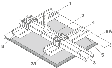
A) Ontkoppelde wandaansluiting
