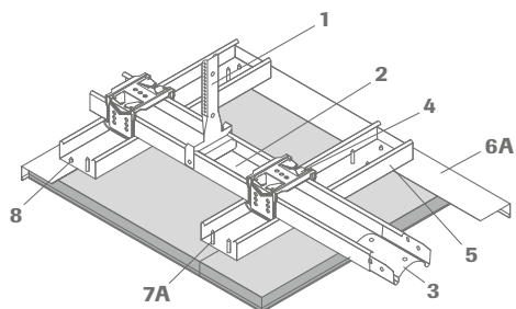
A) Ontkoppelde wandaansluiting
