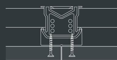
Schroefmontage
