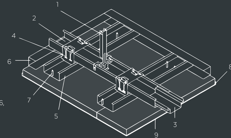
Schroefmontage
