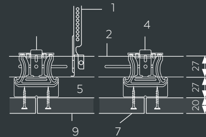
Langsdoorsnede
