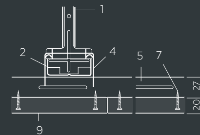
Dwarsdoorsnede
