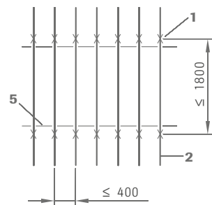
Moduulmaat 1200 x 400 mm
