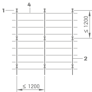
Moduulmaat 1200 x 300 mm
