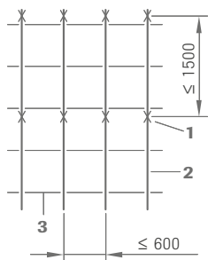
Moduulmaat 600 x 600 mm
